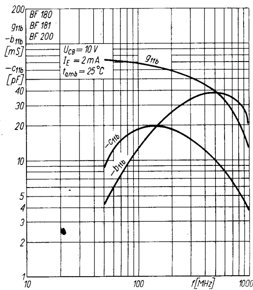
Zależność admittancji wejściowej od częstotliwości g_{11b} ; b_{11b} ; C_{11b} = f(f)
