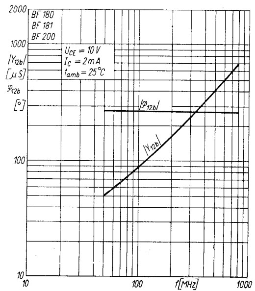
Zależność admittancji przejściowej wstecz od częstotliwości |Y_{12b}| ; \varphi_{12b} = f(f)
