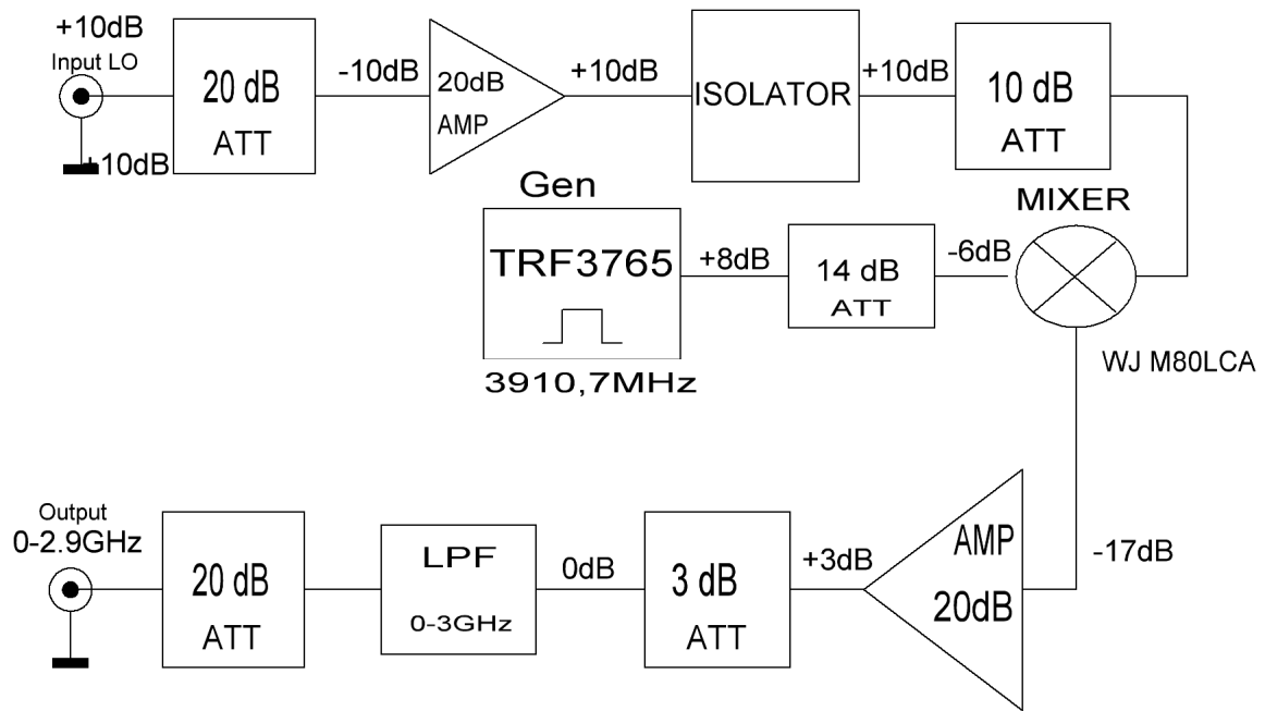
Generator śledzący do HP-8561E
