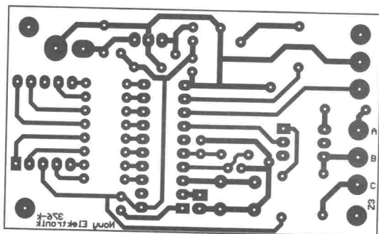
376-k Sterownik do zgrzewarki
